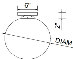
Classic mounting / Montage classique
